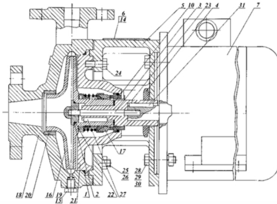
Разрез насоса XM2/25
